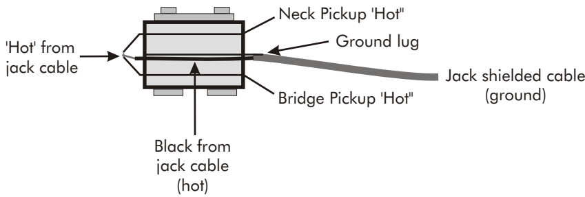
Volume pot wiring:
